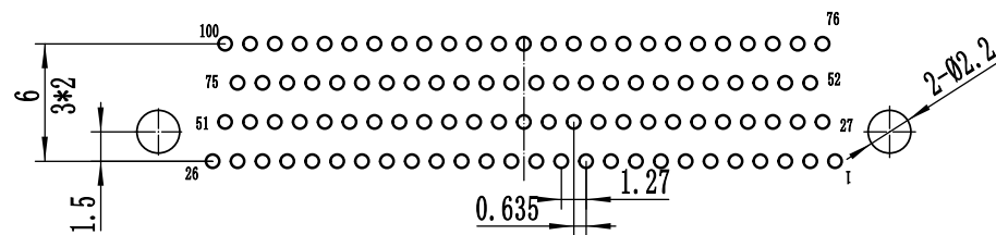
PCB开孔尺寸图
